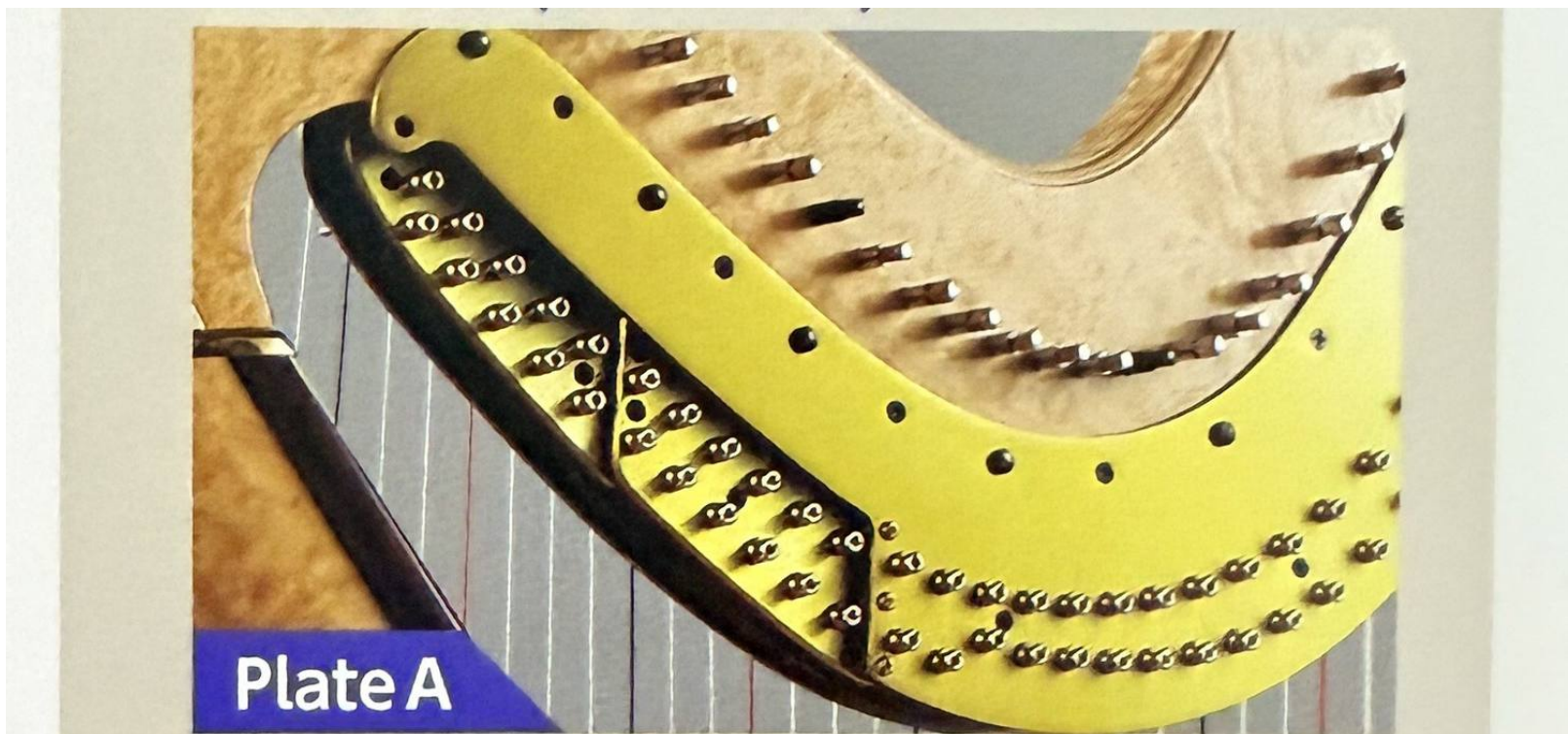
Plate A（弦軸板 A 型） 適用型號：47S-Ex／47D-Ex／47C-Ex
